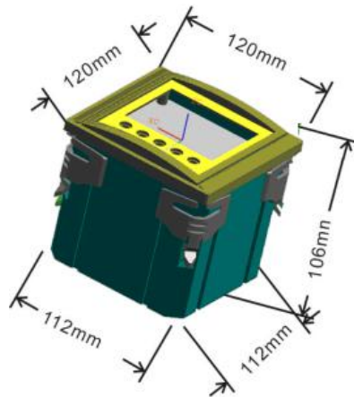
图1 控制器尺寸示意图
