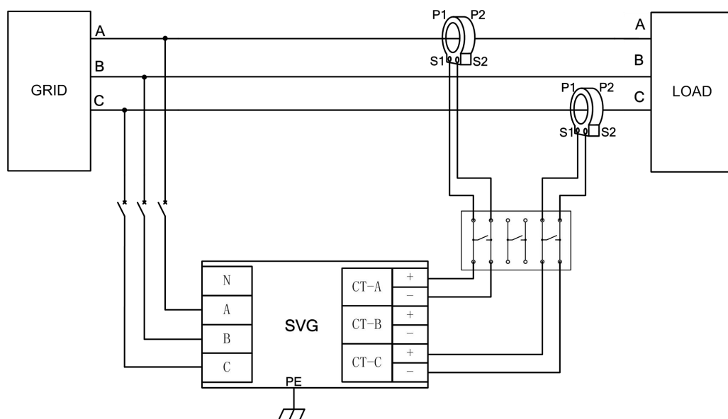
图 3-2 三相三线制
