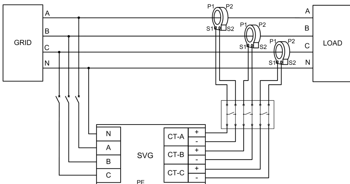
图3-1 三相四线制
