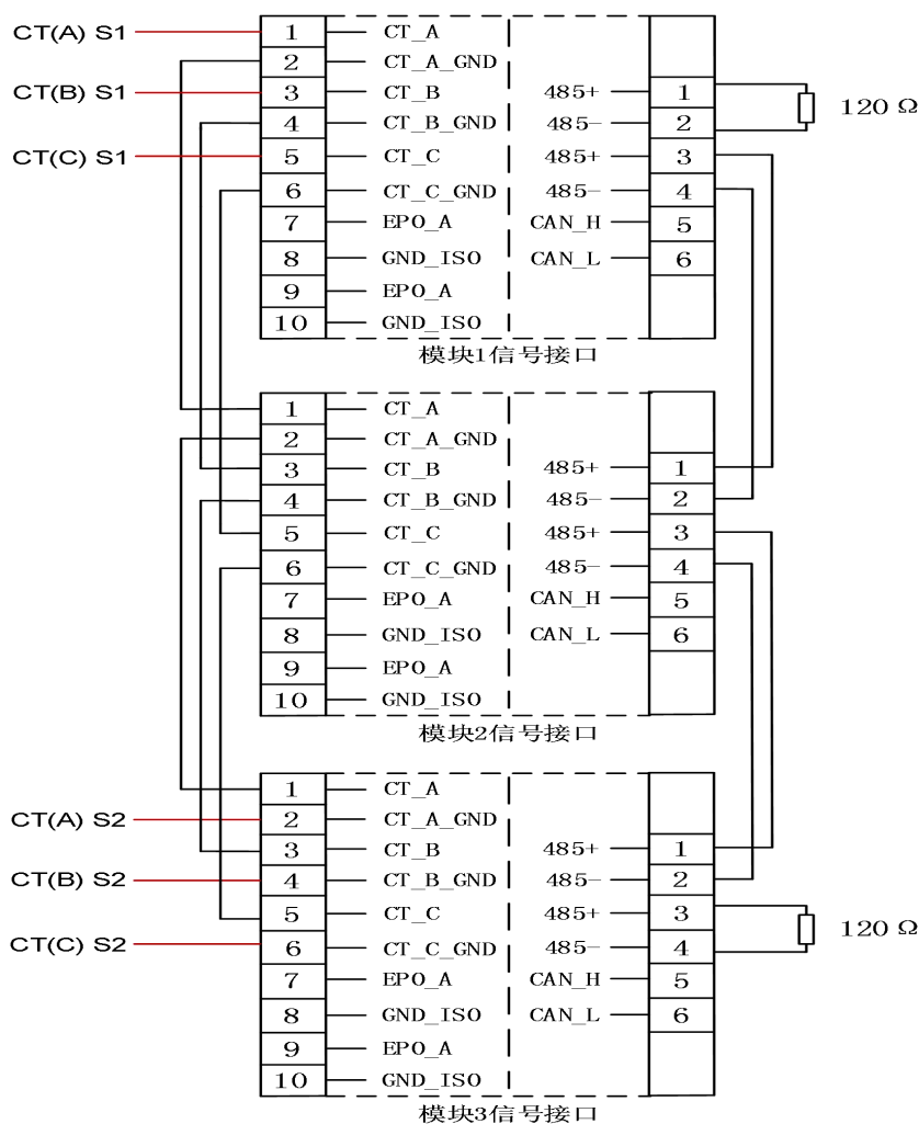
图 3-5 多模块 CT 与通信连接示意
